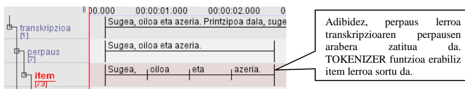
8 Irudia: Tokenizazioa
